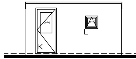
VOORGEVEL BERGING
