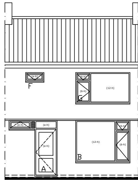
VOORGEVEL
