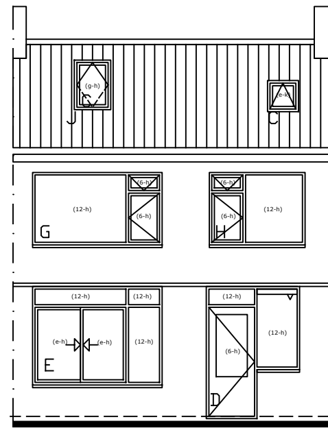
ACHTERGEVEL
