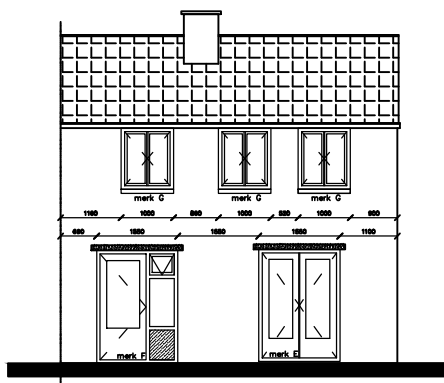
Achtergevels
