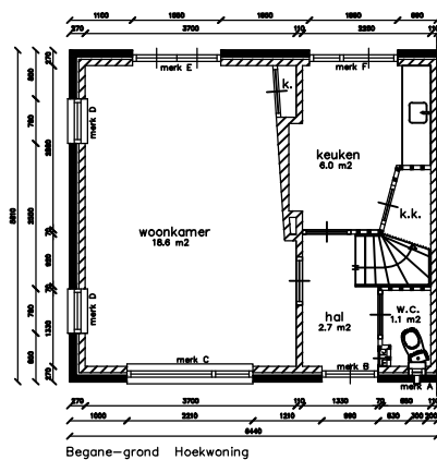
Begane-grond Hoekwoning
