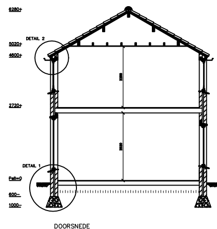
DOORSNEDE
