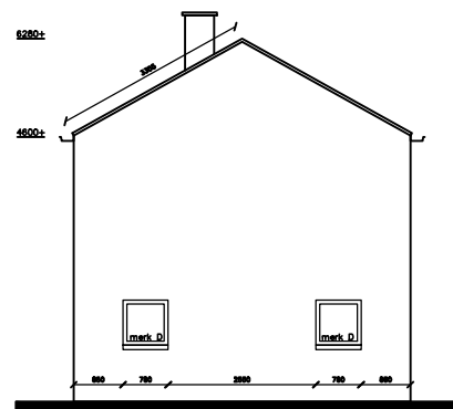
Linker zijgevel
