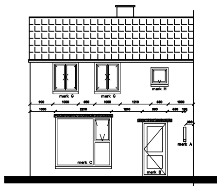
Voorgevels
