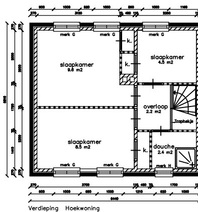
Verdieping Hoekwoning
