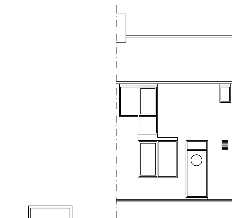
Voorgevel
