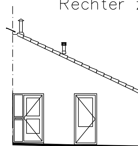
Kopgevel
