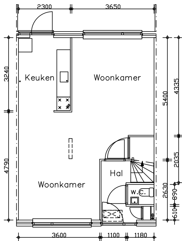
Begane grond
