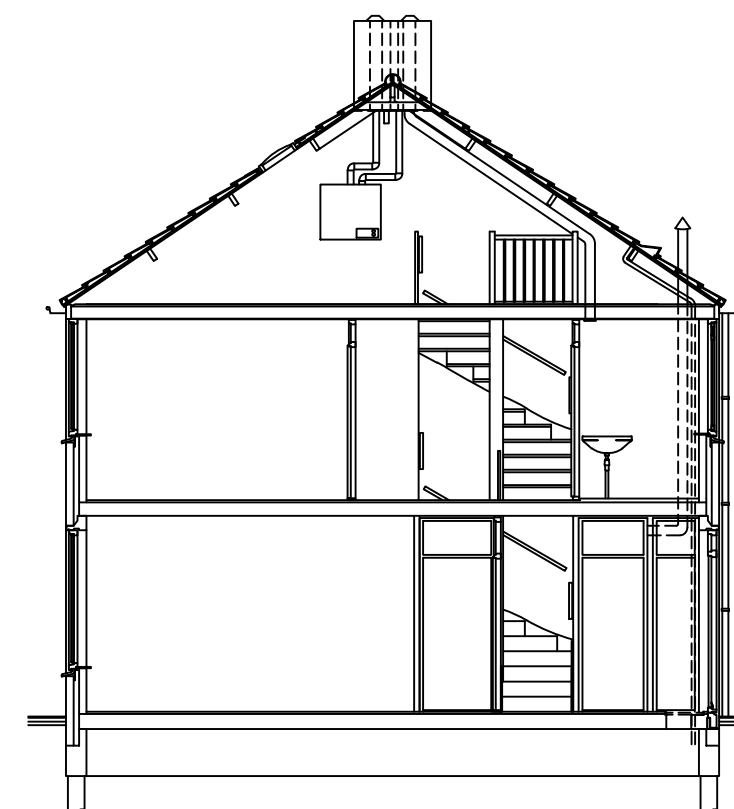
Doorsnede
