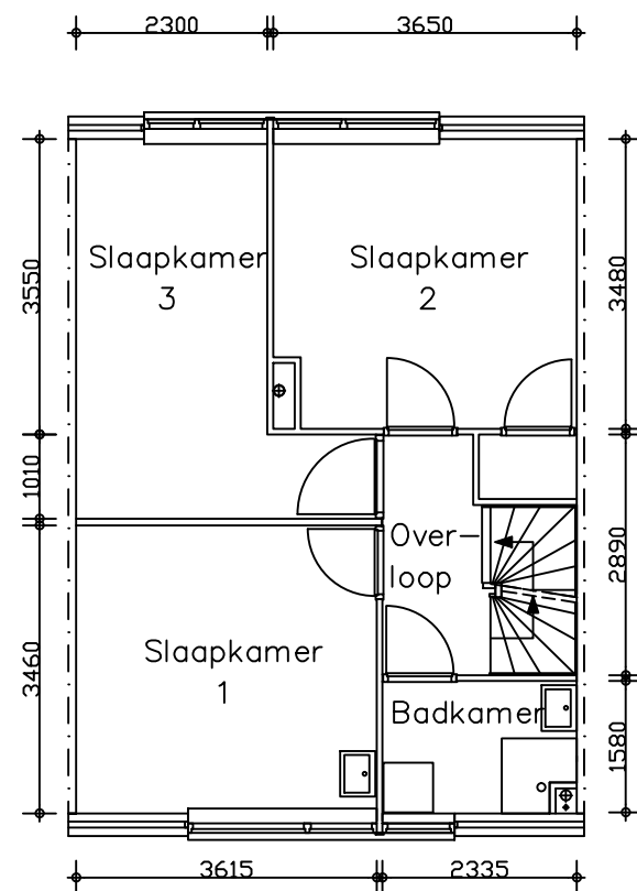
Verdieping
