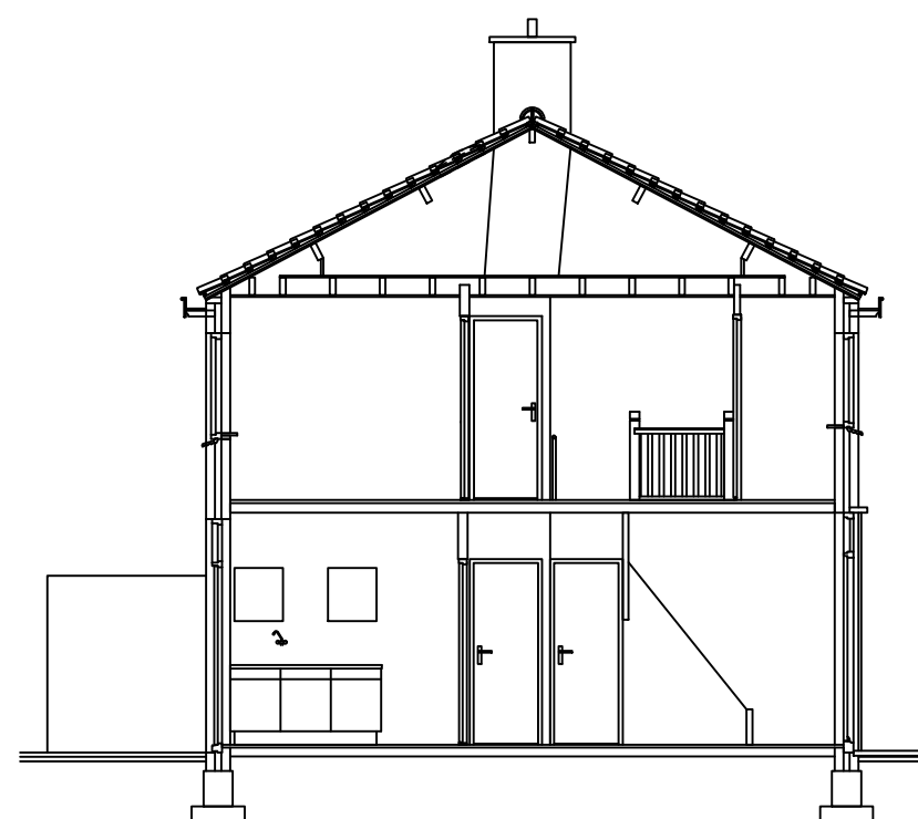
Doorsnede
