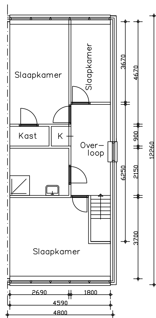
Verdieping
