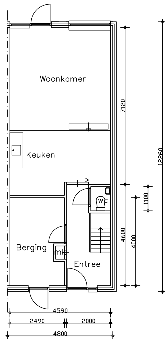
Begane grond
