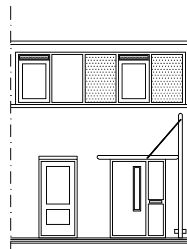
Voorgevel
