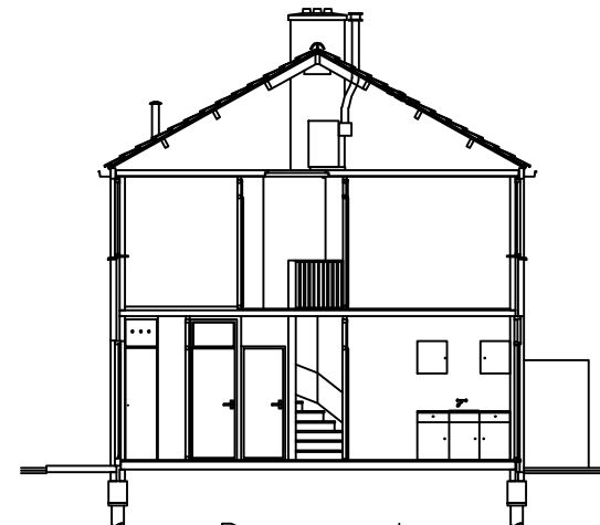
Doorsnede
