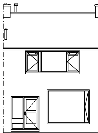
Voorgevel
