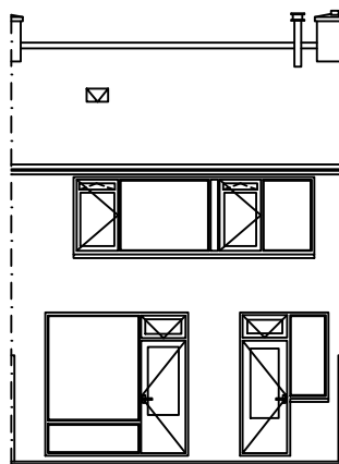
Achtergevel
