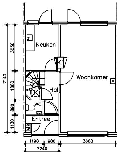
Beganegrond
