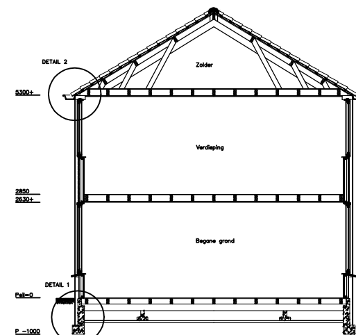
Doorsnede A-A
