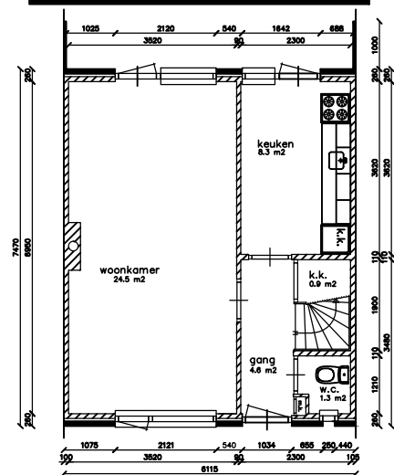
Tussenwoning
