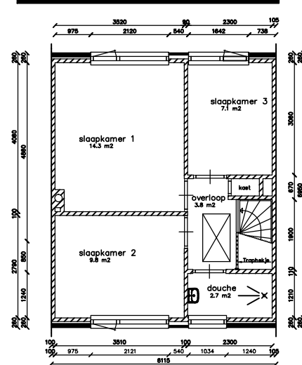
Tussenwoning verdieping
