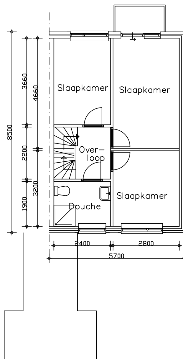
Verdieping
