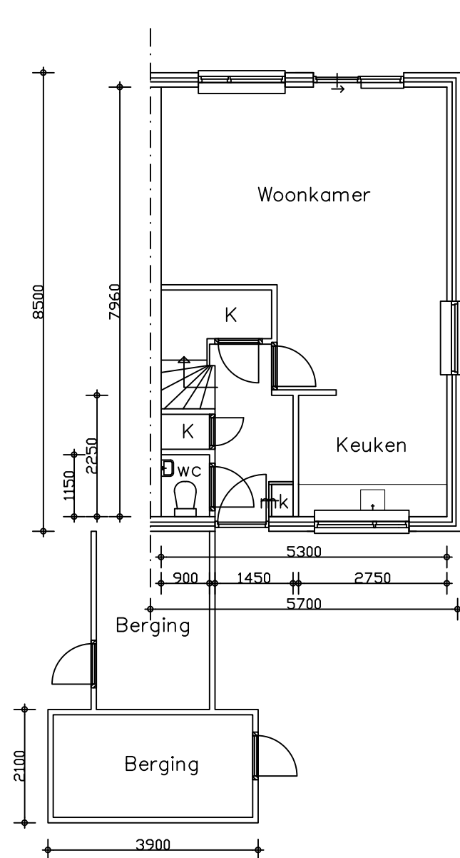
Begane grond
