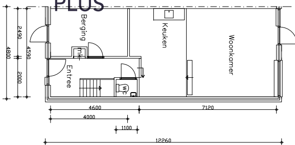
Beganegrond
