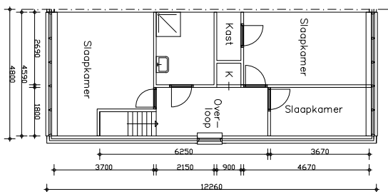
Verdieping
